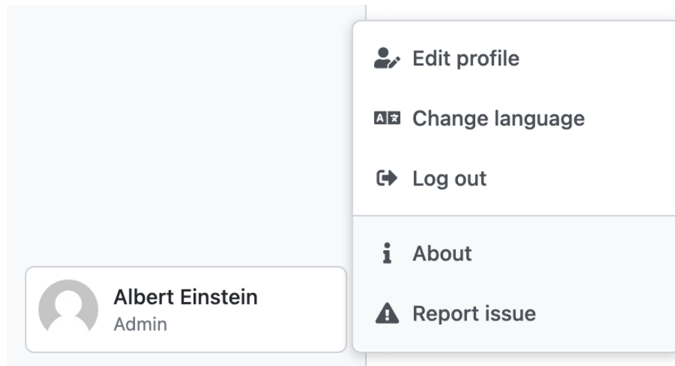
Fig. 76: Profile menu.
